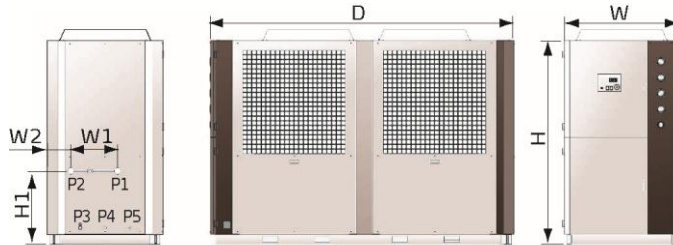
SIC-48A-R2~SIC-75A-R2
